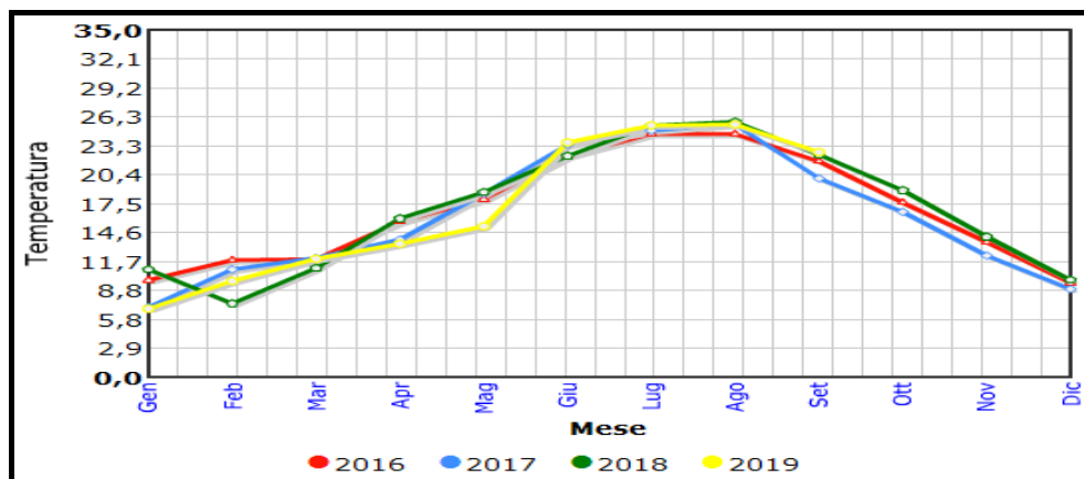
Figura n. 7: andamento medio della temperatura negli anni di riferimento (elaborazione Arsiat)
