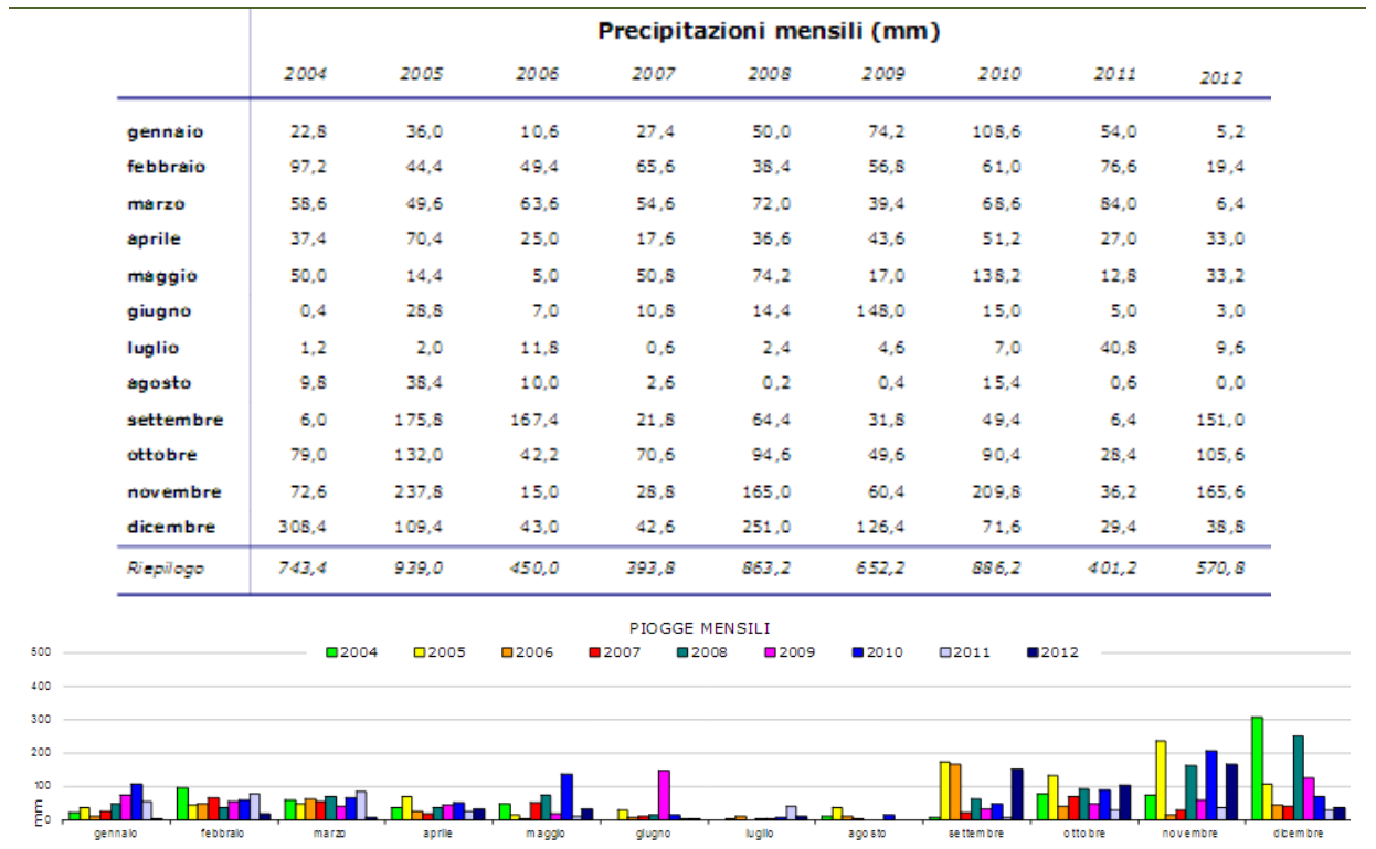
Figura n. 6: precipitazioni mensili (elaborazione Arsiat)
