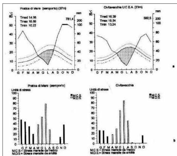
Figura n. 18: diagrammi Bagnouls-Gaussien (a) e Mitrakos (b) delle stazioni pluviometriche relative all'unità fitoclimatica 13 (da Carta del Fitoclima del Lazio, Assessorato Agricoltura e Foreste, Caccia e Pesca della Regione Lazio , 1994)
