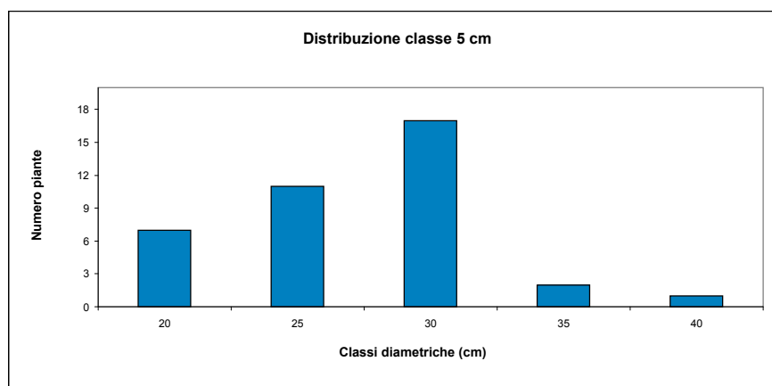
Grafico n. 2: distribuzione diametrica dell'area di saggio n. 6
