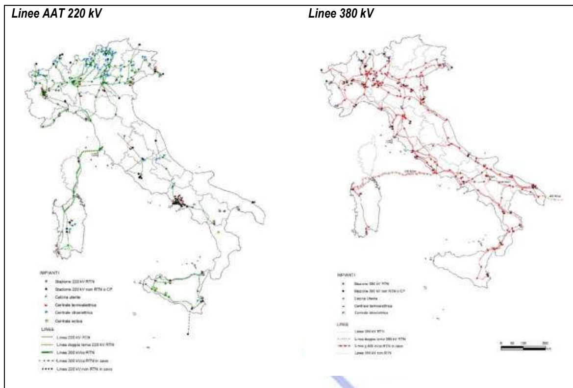
Fig. 7 – Estensione della rete di distribuzione elettrica ad AAT (220 kV e 380 kV) in Italia
