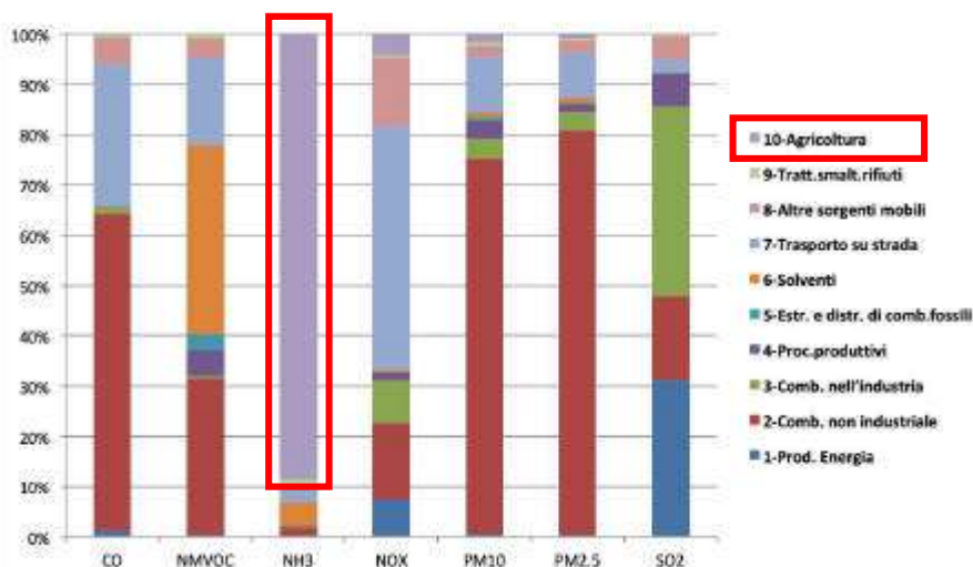
Figura 3-69 Inventaria LAZIO2015 vers.2019: contributi percentuali dei diversi macrosettori alle emissioni totali regionali.
