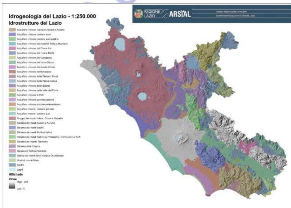
Tavola A-1.e Idrogeologia
