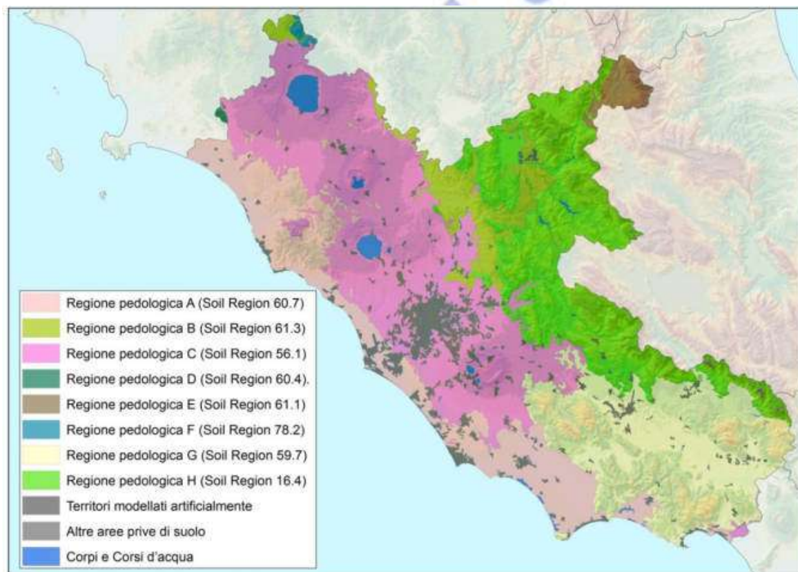
Figura 3 Regioni pedologiche del Lazio
