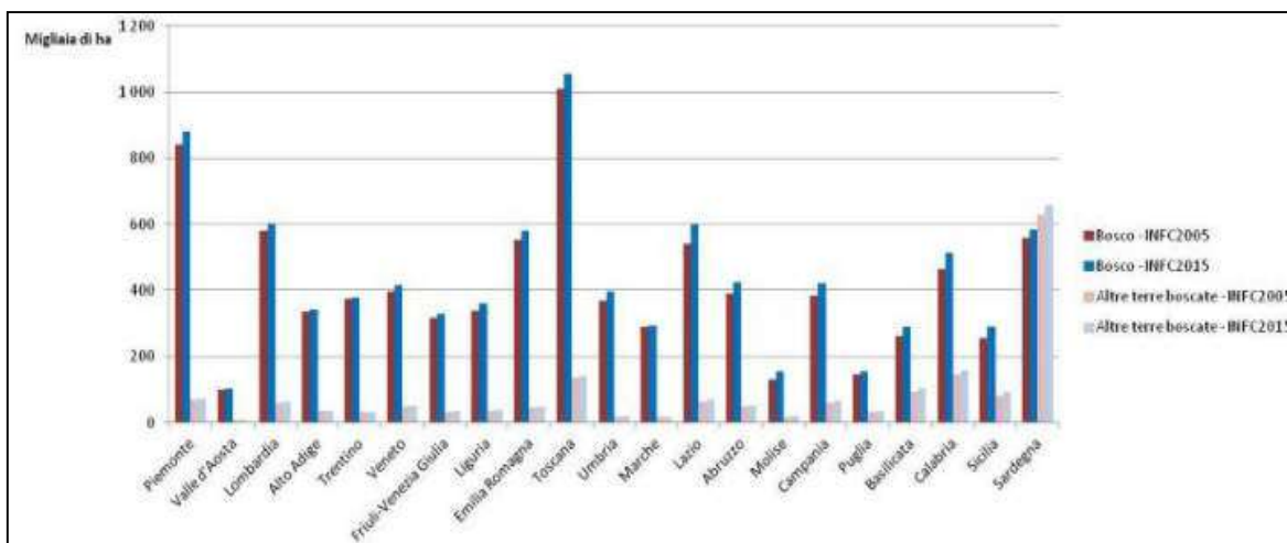
Fig.14 – Stime di superficie da INFC2005 e proiezioni di superficie per INFC2015 del bosco e altre terre boscate esclusi impianti di arboricoltura 4
