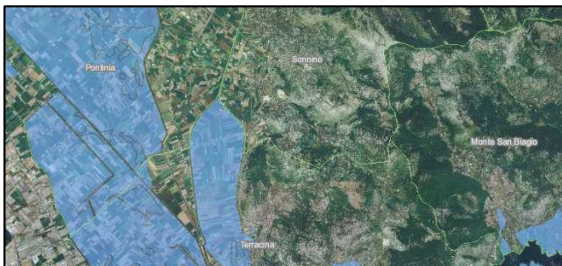
Tavola A3 1 3 Pericolosità idrogeologica
