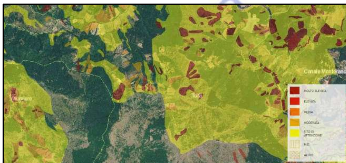
Esempio da Tavola A3 1 2 PAI Pericolosità da frana
