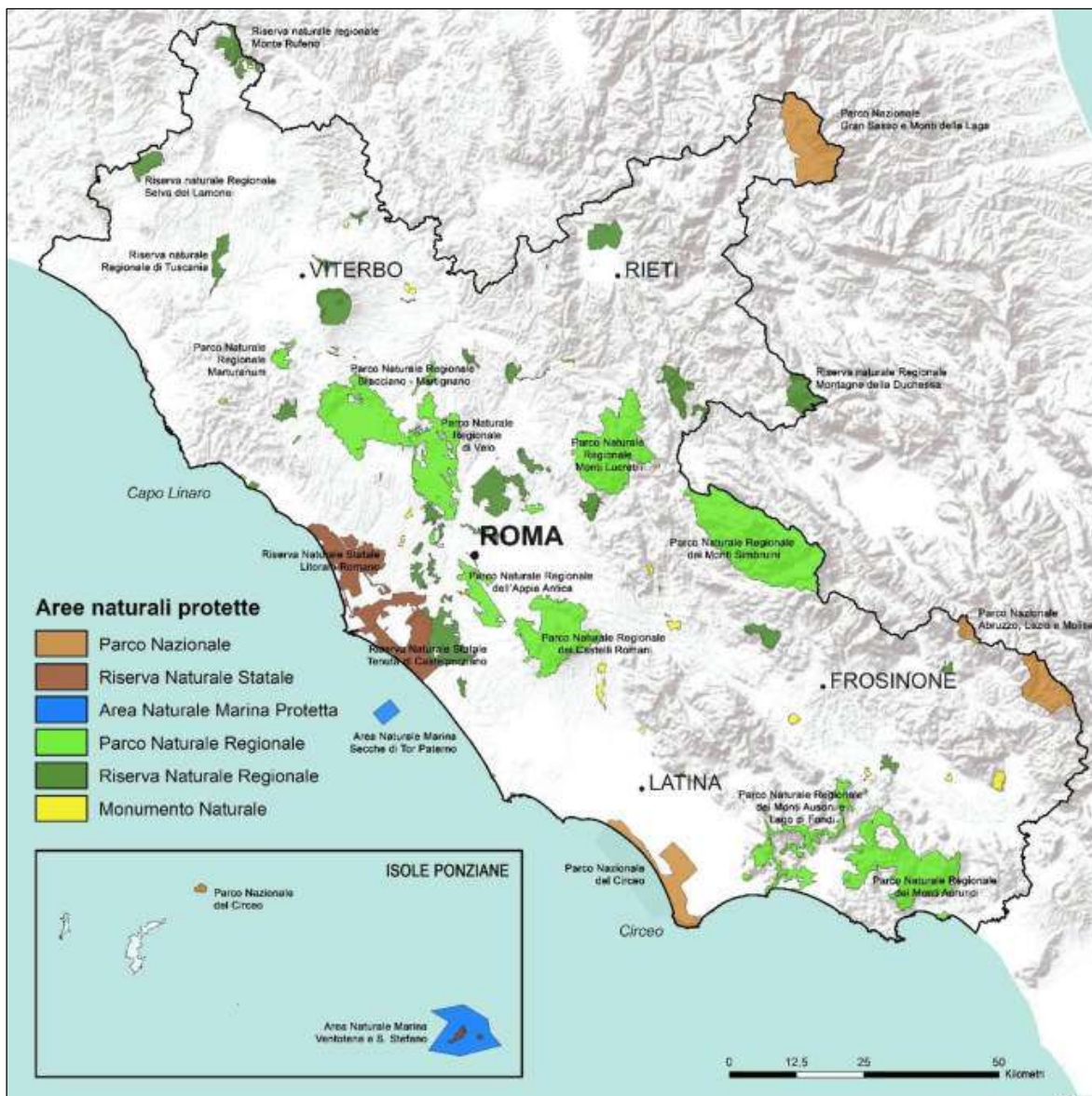
Fig. 2. Sistema delle aree naturali protette della Regione Lazio per tipologia di area protetta
