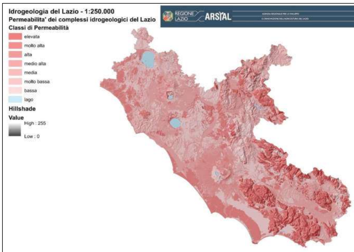
Tavola A-1.f Permeabilit  idrogeologica
