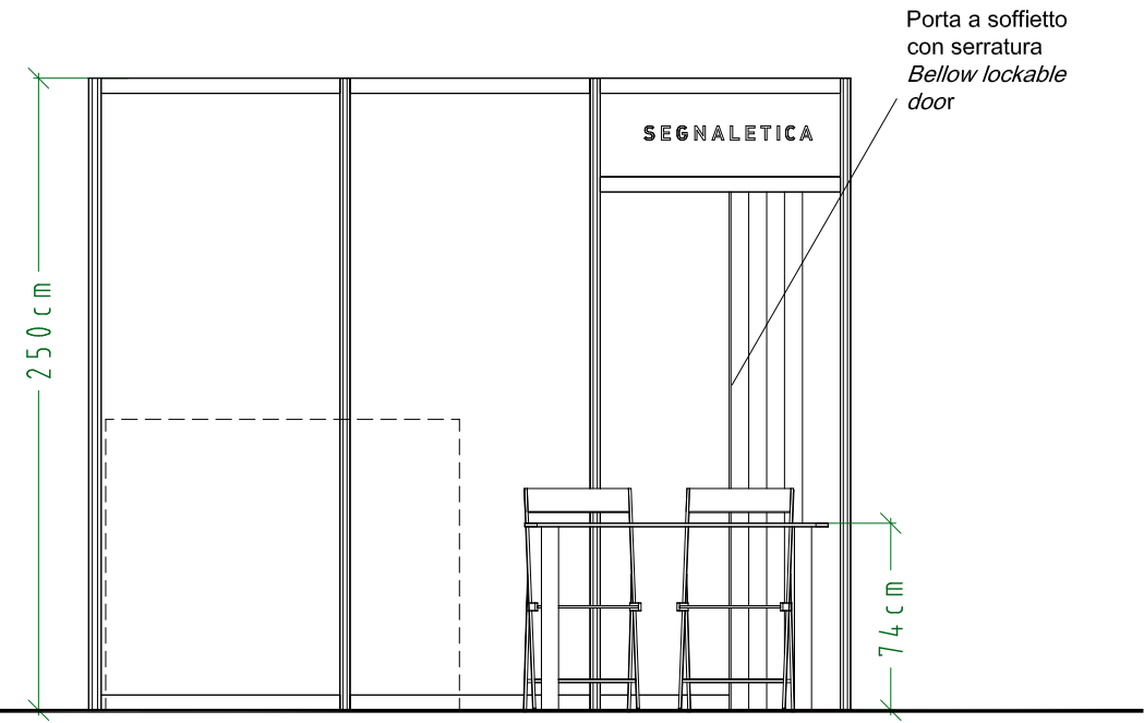
PROSPETTO/FRONT ELEVATION
