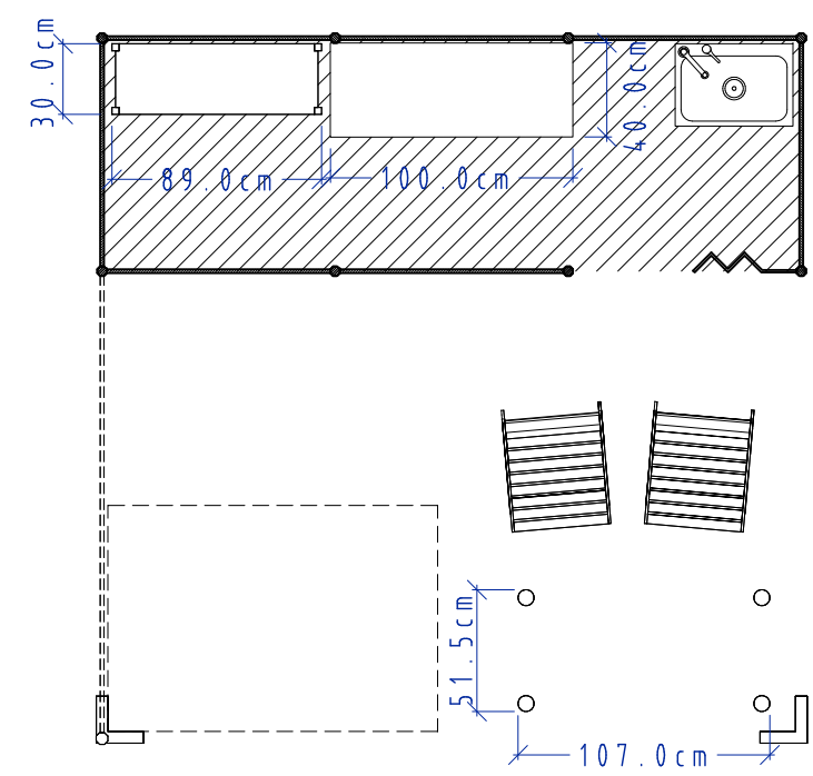
PLANIMETRIA (sezione h.60cm) PLAN (section h.60cm)
