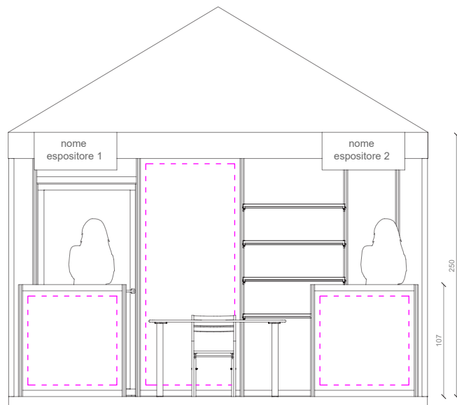
PROSPETTO/ FRONT ELEVATION
